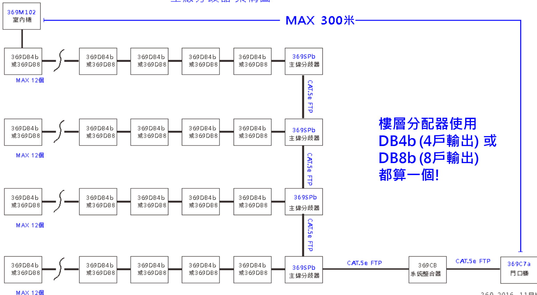
主線分歧器 架構圖
